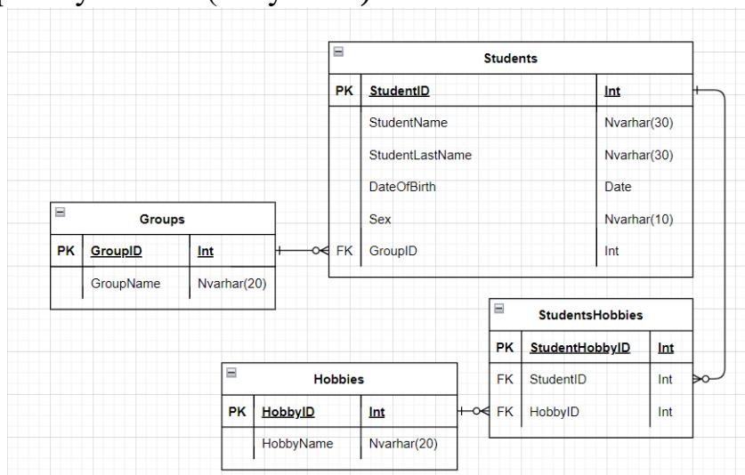
Рисунок 4 – ER-диаграмма
