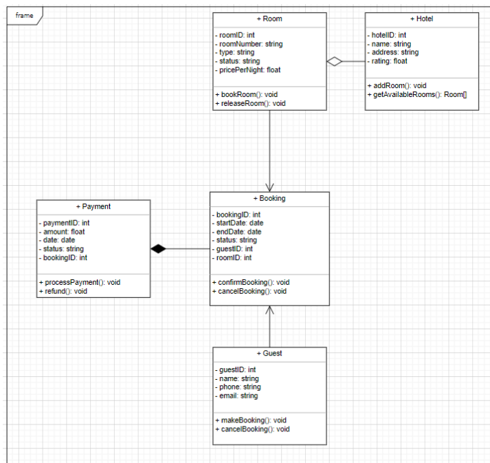
Рисунок 1 – Диаграмма классов
