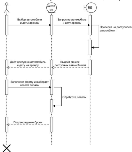
Рисунок 2 – Диаграмма последовательностей
